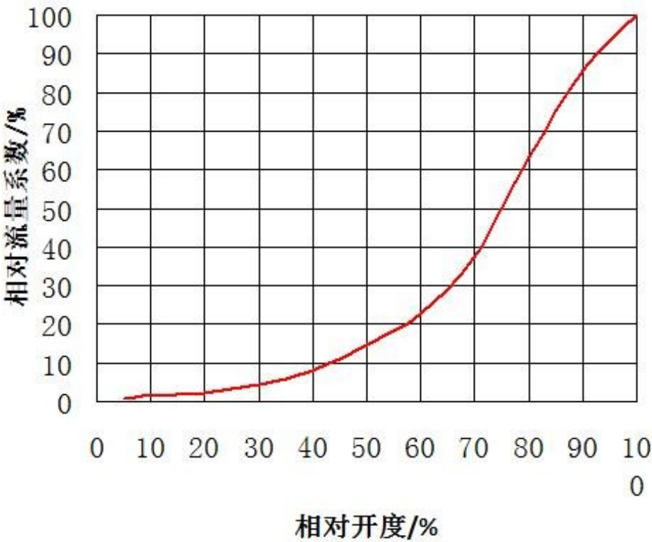
4、固有流量特性曲线
